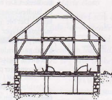
Prinsippskisse av en enhetslåve som ligner driftsbygningen på Nordre. Vi ser den langsgående låvebrua øverst med rom under og til sides for fôrlagring. I 1. etasje fjøs med møkkakjeller under. På Nordre Østensjø er det stall og fjøs i nordenden, redskapslager i sørenden. I midtseksjonene og i hele 2. etasje er det förlager. Illustrasjon fra "Akershusiske låver 1870-1970".
