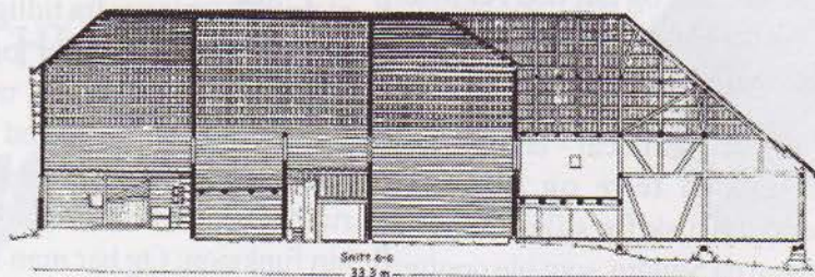
Snitt-tegning gjennom driftsbygningen på Søndre. Den høyre delen ble tilbygget seinere i bindingsverk. Legg merke til takkonstruksjonen med laft helt opp til mønet.
